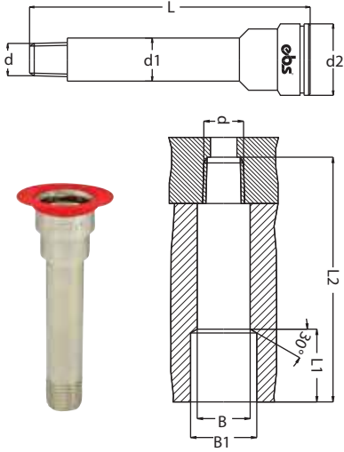
Erkek Uzatma Uçlar / Extension
