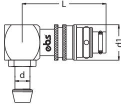
90° Hortum Gövde / 90° Hose Tail Socket
