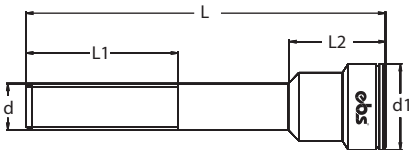
Erkek Uzatma Uçlar / Extension
