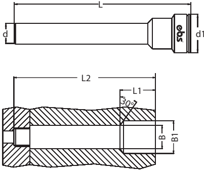
Erkek Uzatma Uçlar / Extension
