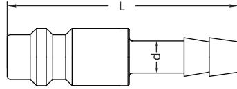
Hortum Uç / Hose Plugs
