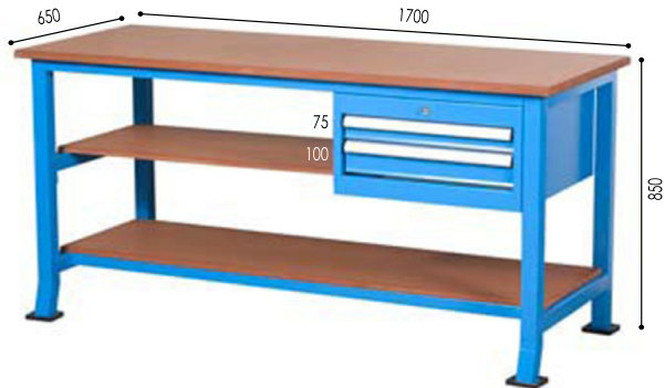
3705 İki Çekmeceli Panosuz Çalışma Masası
