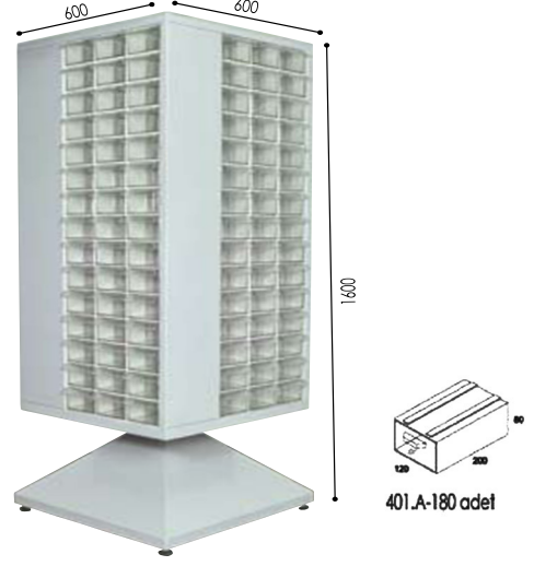
ÇKTS 401 154 Çekmeceli Stand
