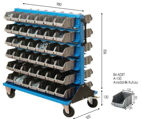
4089 Çift Yönlü Avadanlık Arabası
