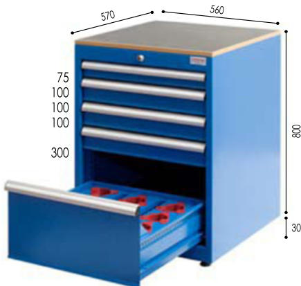
2650 5 Çekmeceli Takım Dolabı (1 CNC Çekmeceli)
